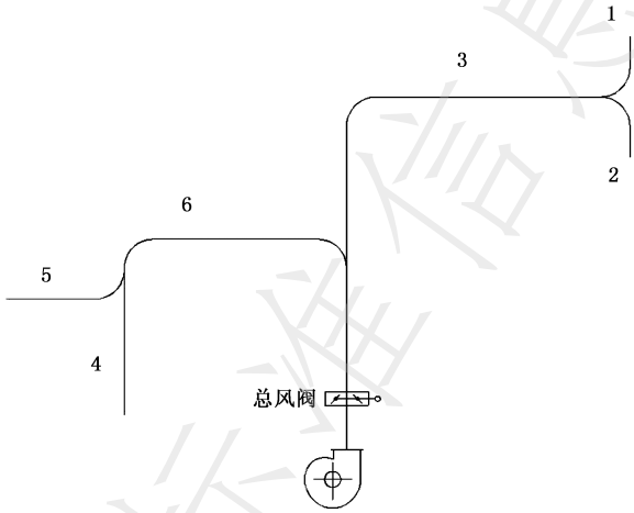
图 D.2 流量等比分配法管网风量平衡图
