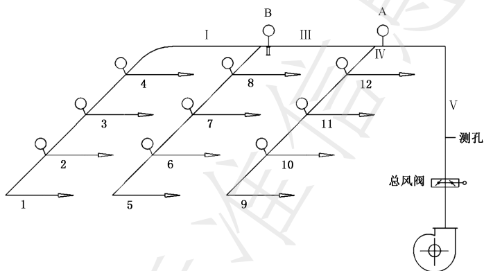
图 D.3 系统风量平衡调节示意图
