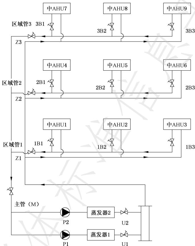
图 C.2.2-2 设备管路平衡后采用“中 AHU”
