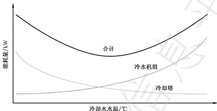
图 E.2-2 冷却水温度对制冷系统能耗影响示意图
