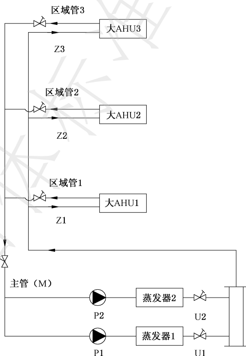
图 C.2.2-3 支管路平衡后采用“大 AHU”
