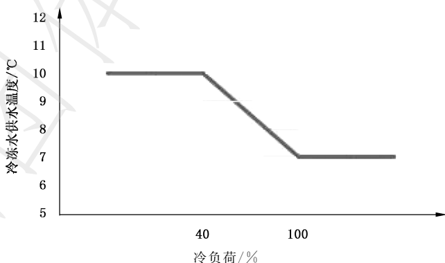
图 E.1.2 基于建筑冷负荷的冷冻水变供水温度控制逻辑
