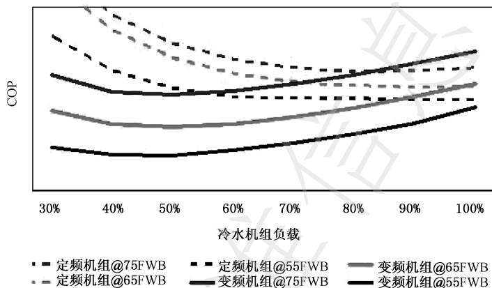
图 E.3.1 制冷机效率与负荷率关系曲线图
