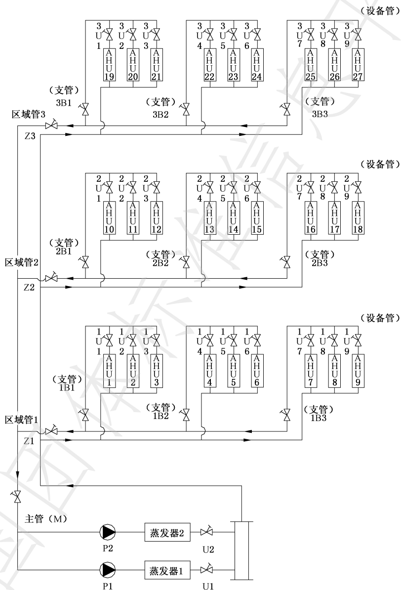
图 C.2.2-1 分区空调冷冻水系统图
