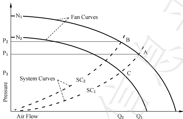
图 F.2.1 风机性能曲线与管路特性曲线关系图
