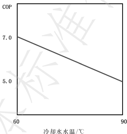
图 E.2-1 冷却水温度对冷水机组 COP 影响示意图
