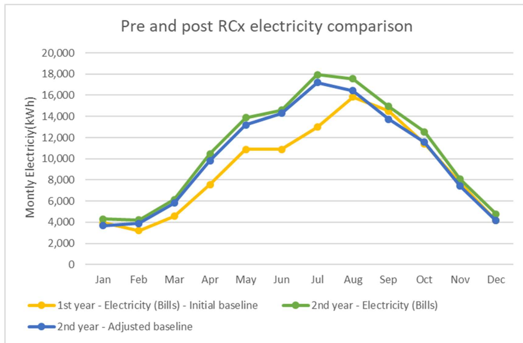
圖 4.5(c)回歸調整後電費比較
