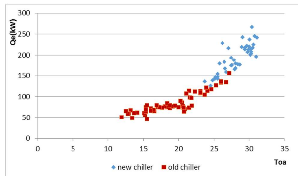
圖 A.2(b)冷負荷與室外環境溫度比對（重新校驗前）
