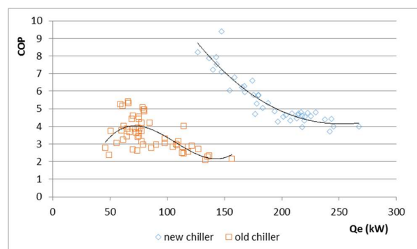
圖 A.2(c)冷水機 COP 與冷負荷比對（重新校驗前）
