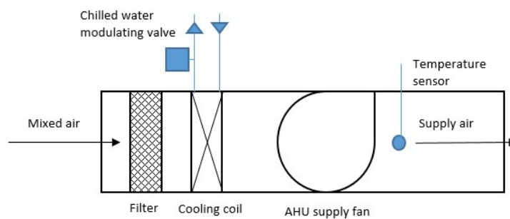
圖 4.2.5(e)送風機數據點位置示意圖
