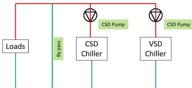
圖 A.3(a)冷水機組簡單框圖
