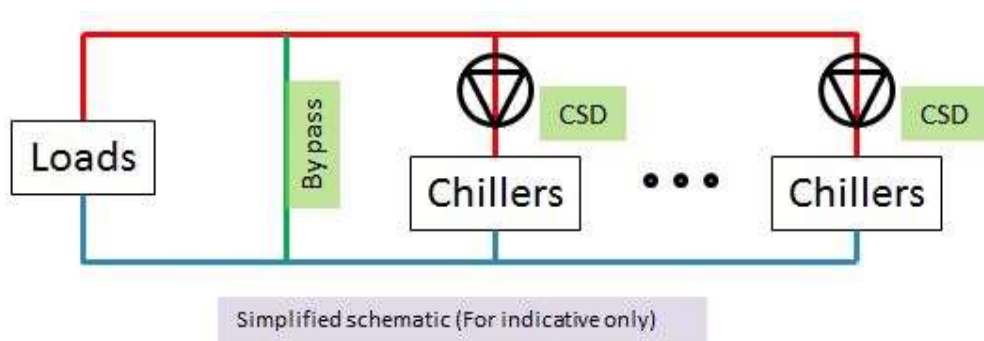
圖 A.4(a) 冷水機組簡單框圖
