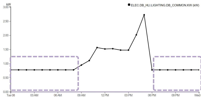
圖 4.2.5(i)照明超時操作數據示例
