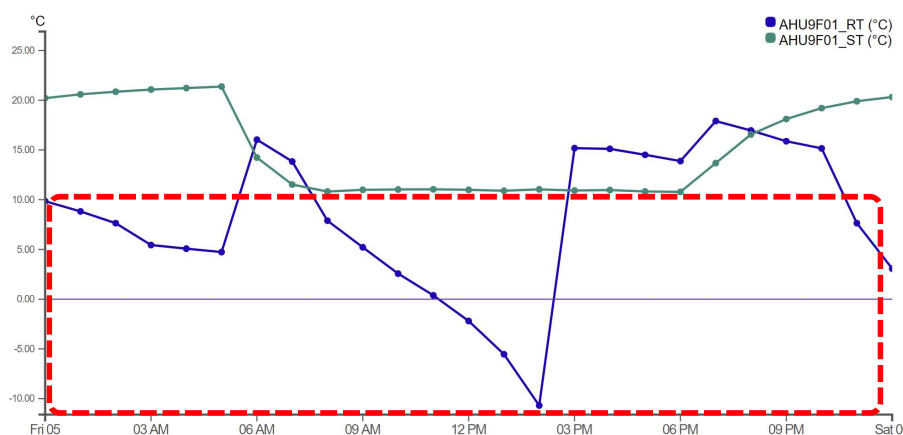
圖 4.3.1(b)溫度超出範圍數據示例
