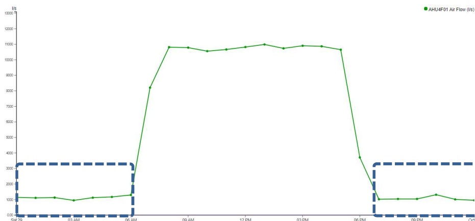
圖 4.2.5(f)送風機超時操作數據示例
